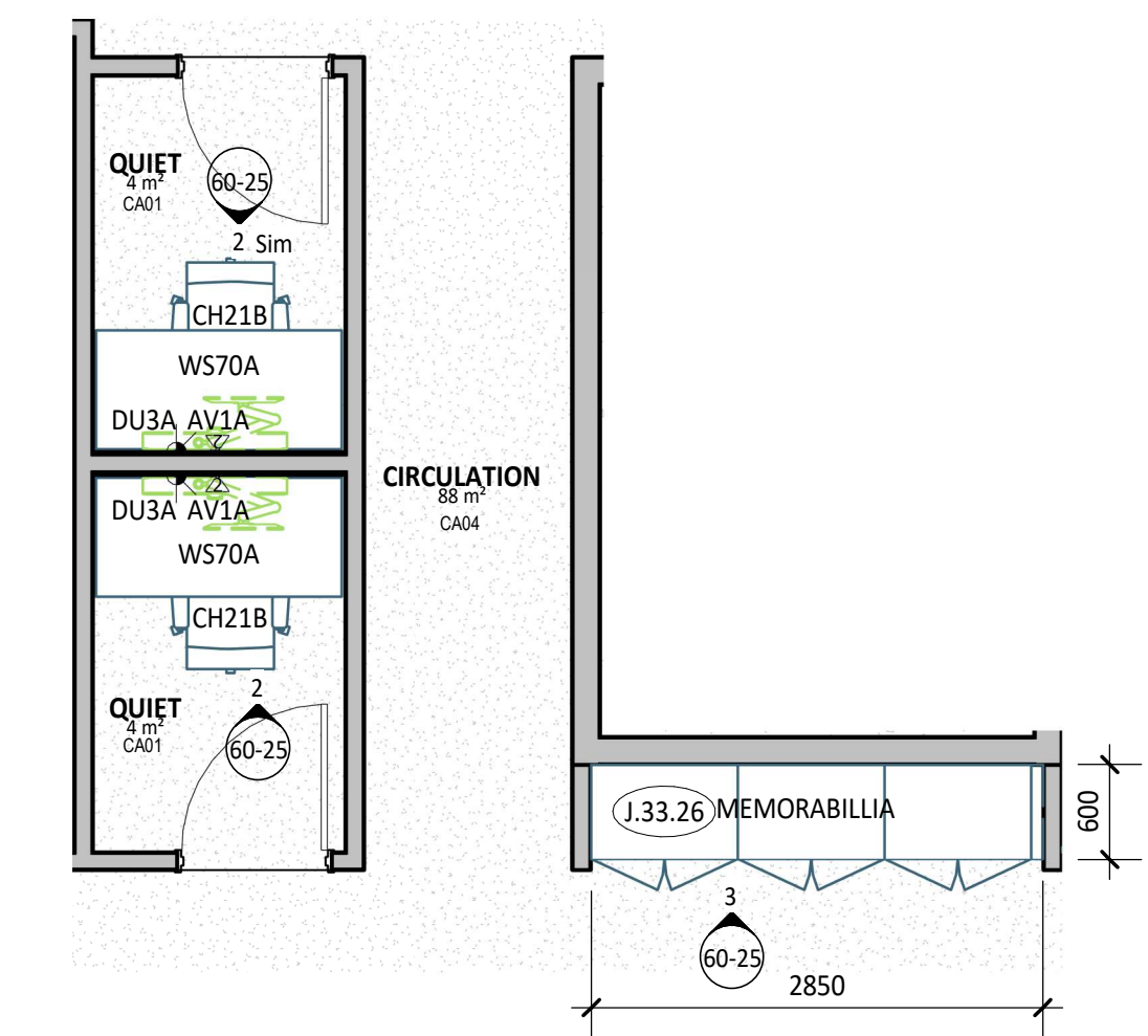
1 PLAN DETAIL 1 : 50
