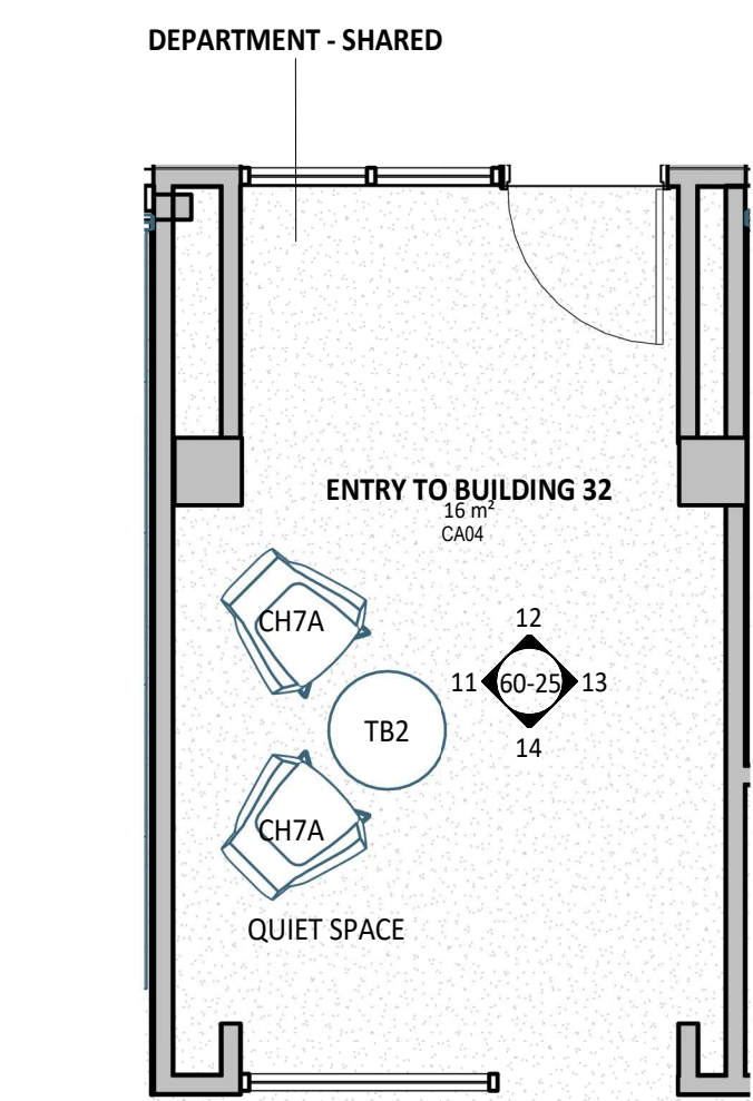
10 PLAN DETAIL 1 : 50
