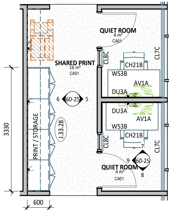
4 PLAN DETAIL 1 : 50
